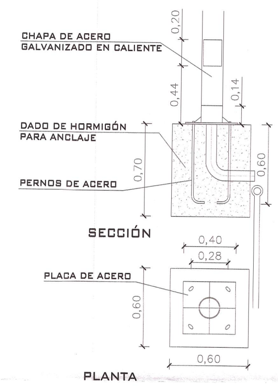
DETALLE ANCLAJE DE BACULO 7.00M
