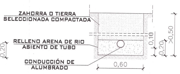
CONDUCCIÓN DE ALUMBRADO
