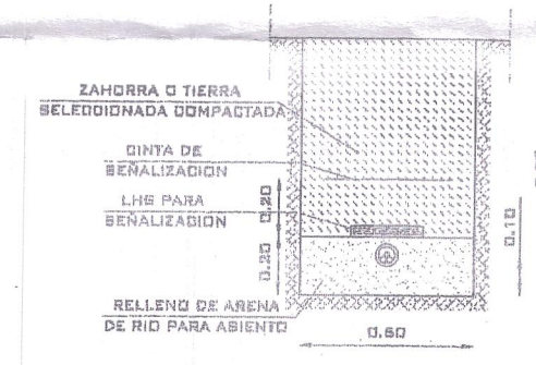
CONDUCCION DISTRIBUCION EN ALTA TENSION ENTERRADA
