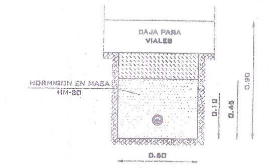
CONDUCCION DISTRIBUCION EN ALTA TENSION ENTERRADA
