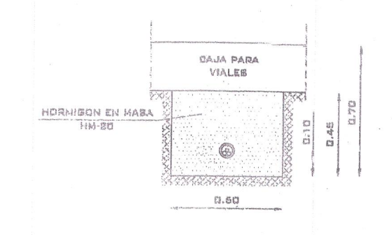
CONDUCCION DISTRIBUCION EN ALTA TENSION ENTERRADA
